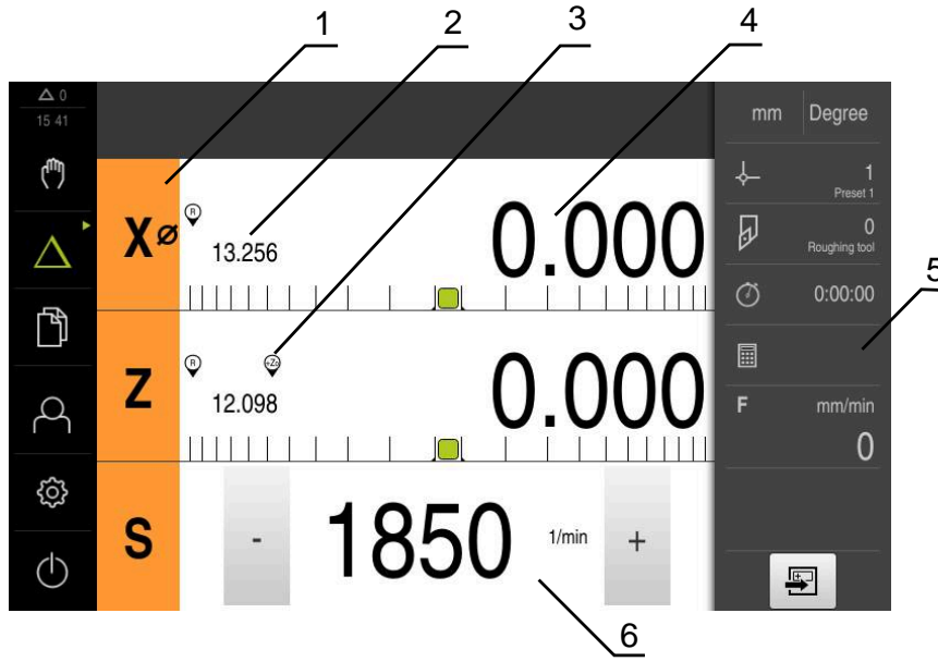
Şekil 15: MDI işletimi menüsü
