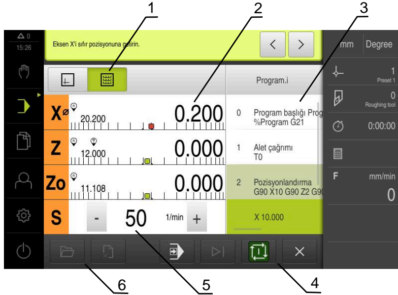
Şekil 45: Program akışı işletim türünde bir program örneği
