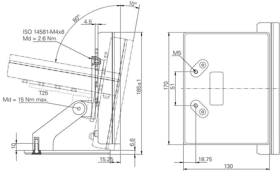
Şekil 59: Multi-Pos ayağıyla cihaz ölçüleri
