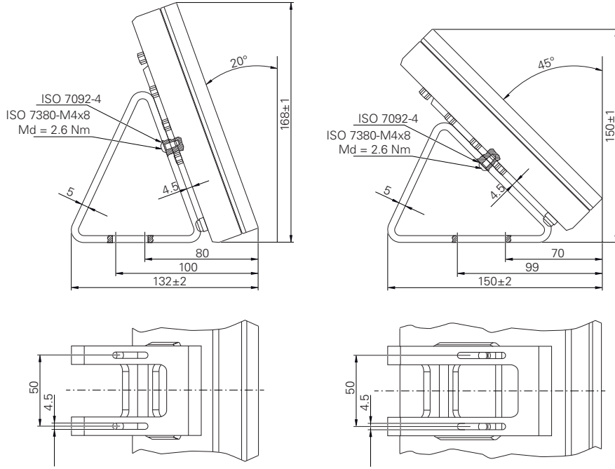
Şekil 58: Duo-Pos ayağıyla cihaz ölçüleri
