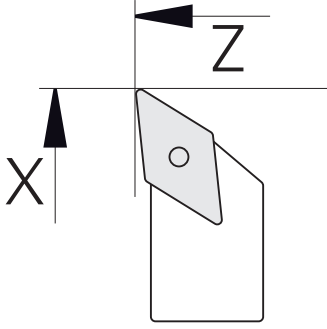
Şekil 30: Perdah keski parametreleri
