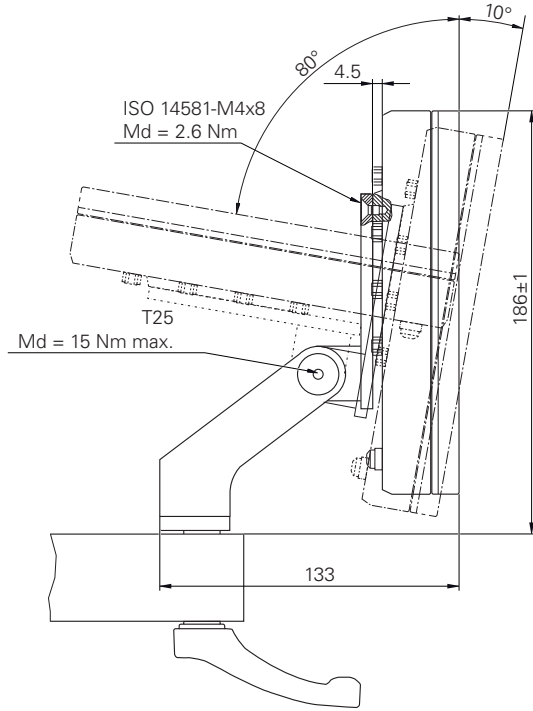
Şekil 60: Multi-Pos tutucuyla cihaz ölçüleri
