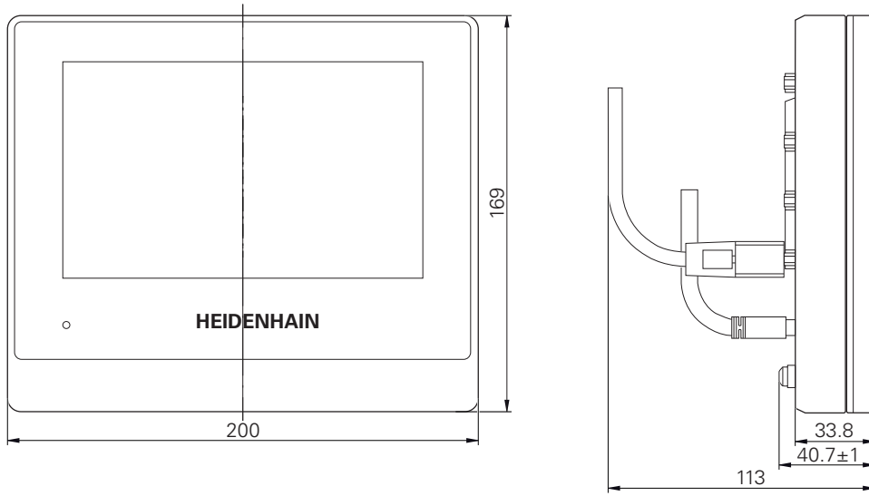
Şekil 53: 1089178-xx kimlik numaralı cihazların gövdesinin ölçüleri
