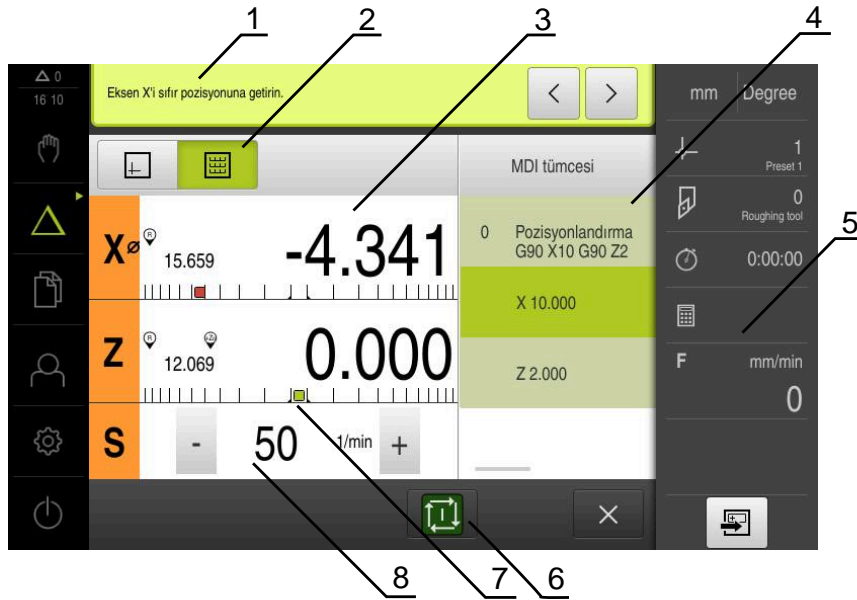
Şekil 40: MDI işletim türünde tümce örneği
