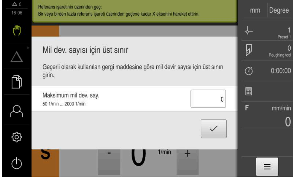
Şekil 37: Mil dev. sayısı için üst sınır diyalogu
