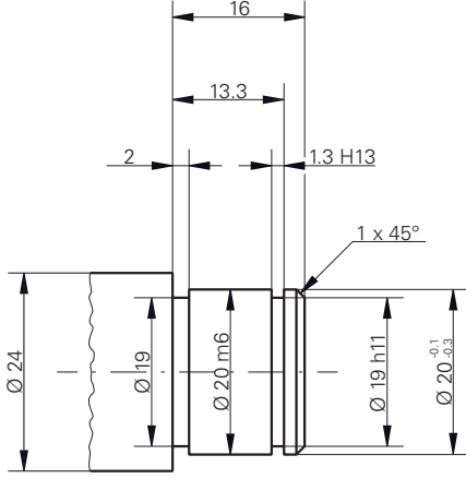
Şekil 29: Örnek malzeme – Teknik çizim
