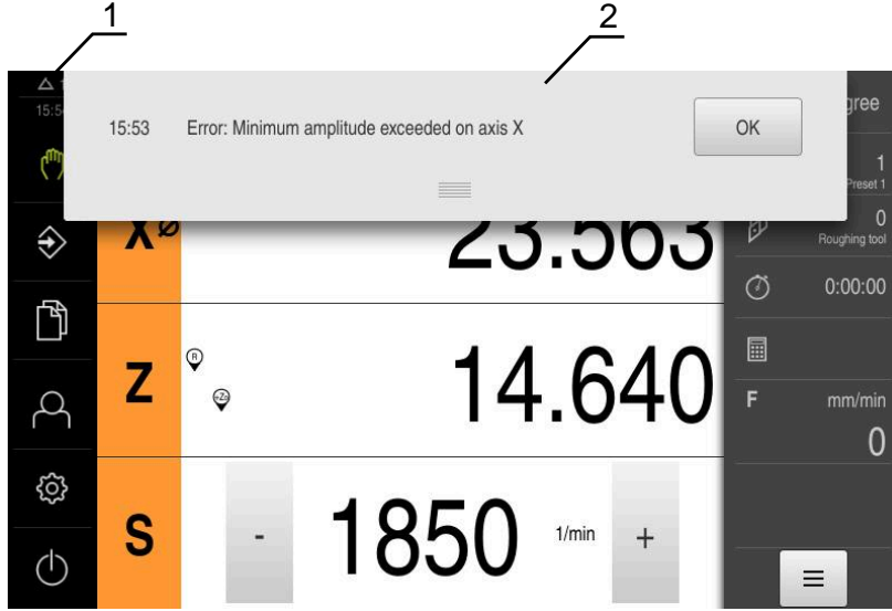
Şekil 23: Çalışma alanında mesajların gösterimi
