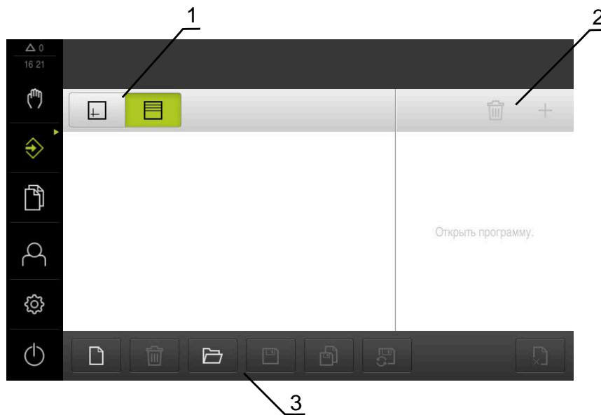
Рисунок 9: Меню Программирование
