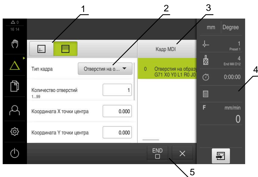
Рисунок 7: Диалоговое окно Кадр MDI
